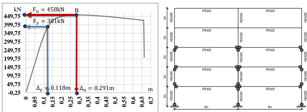
Слика 2. а) Распределба на пластични зголбови б) Pushover- крива
