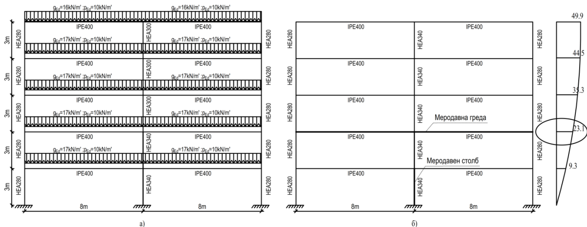
Сл 1. а) Приказ на разгледуваната конструкција б) Хоризонтални поместување од влијание на вкупната проектна сеизмичка сила S_{de} .
