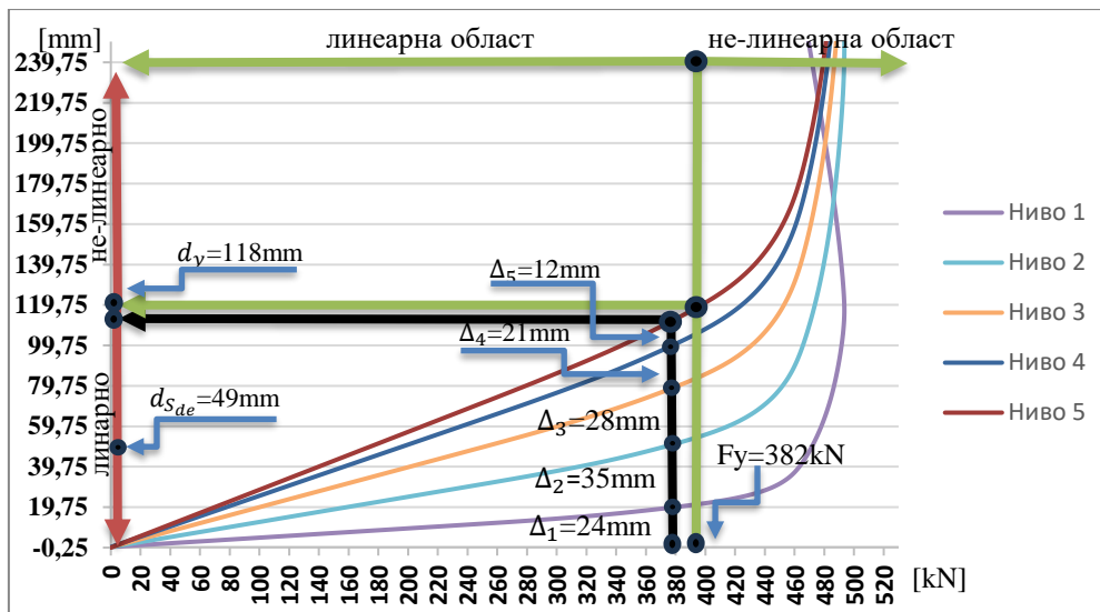
Сл 4. Приказ на хоризонталните поместувања на соодветните нивоа на рамката.
