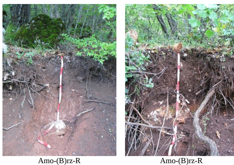
Figure 4. Calcocambisols
