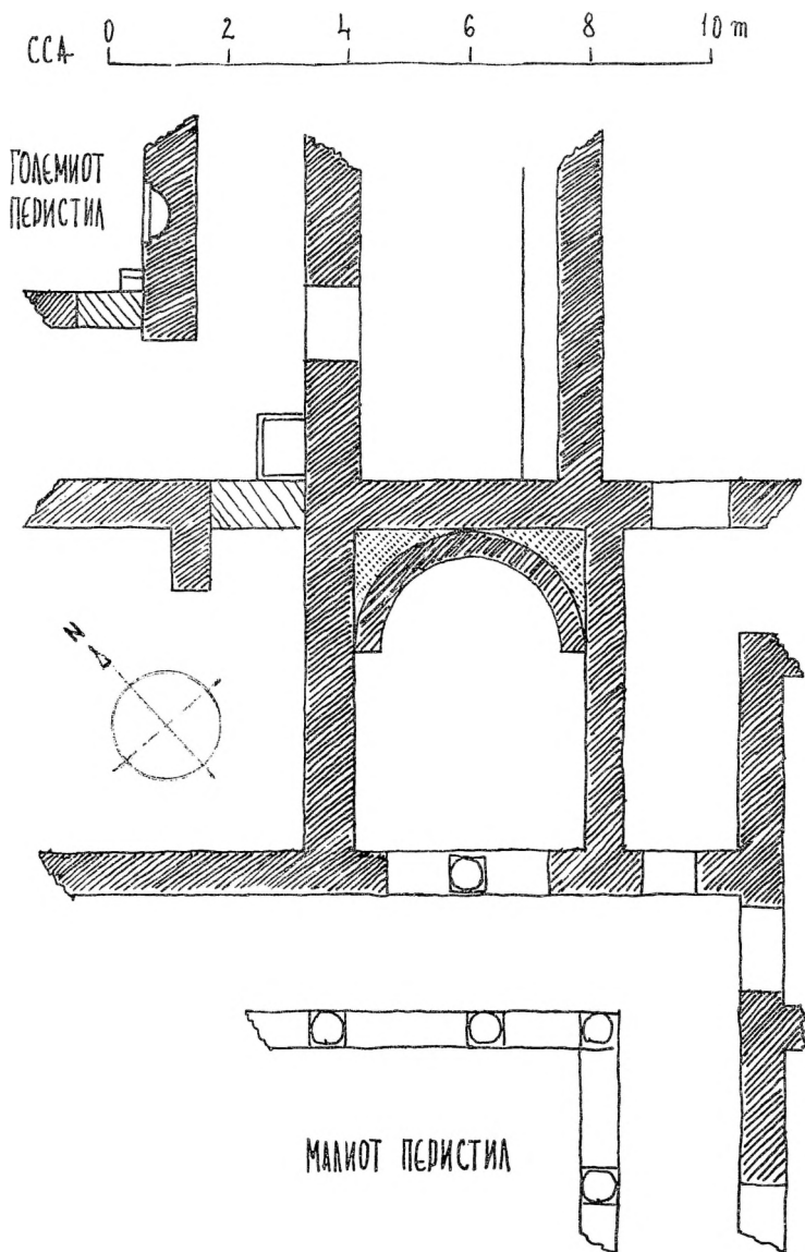
СЛ.12. -МАЛАТА ЈУЖНА АПСИДАЛНА ОДАЈА ВО ПАРТЕНИОСОВАТА ПАЛАТА ВО СТОБИ СЛОБОДНО МЕРНО НАГОЛЕМУВАЊЕ СПОРЕД Б.НЕСТОРОВИЌ И СПОРЕД ДИСПОЗИЦИЈАТА in situ
