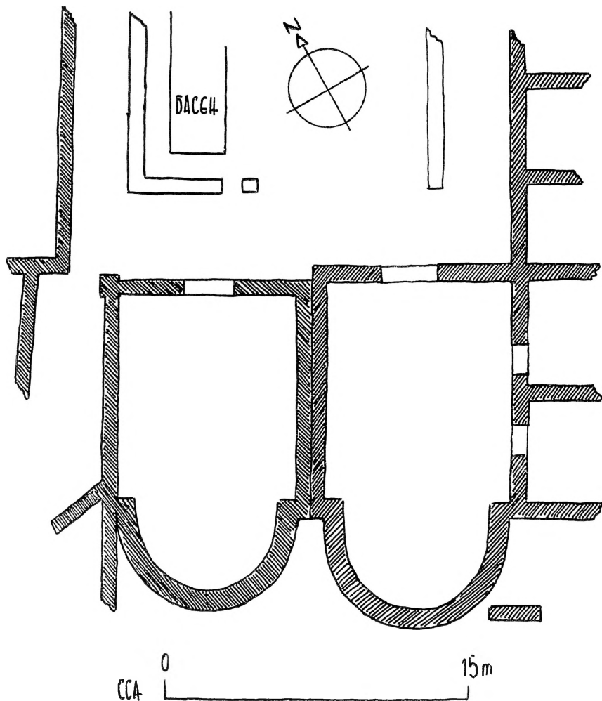
сл. 8 - ДВЕТЕ ГОЛЕМИ АПСИДАЛНИ ДВОРАНИ ВО ПАЛАТАТА ПЕРСИПЕЛИДА СПОРЕД ДИСПОЗИЦИЈАТА IN SITU И СПОРЕД СЛОБОДНО МЕРНО ИСТОПМУВАЊЕ ОД СИТУАЦИОНИОТ ПЛАН НА ИСКОПАНИТЕ ОБЈЕКТИ
