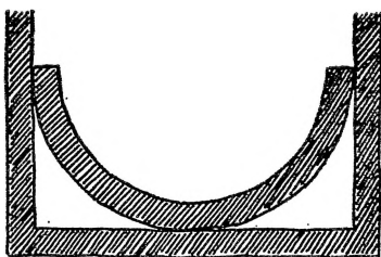
СЛ. 5 - АПСИДАЛНА КОНСТРУКЦИЈА ОД II С ВАРИЈАНТНА ФОРМА
