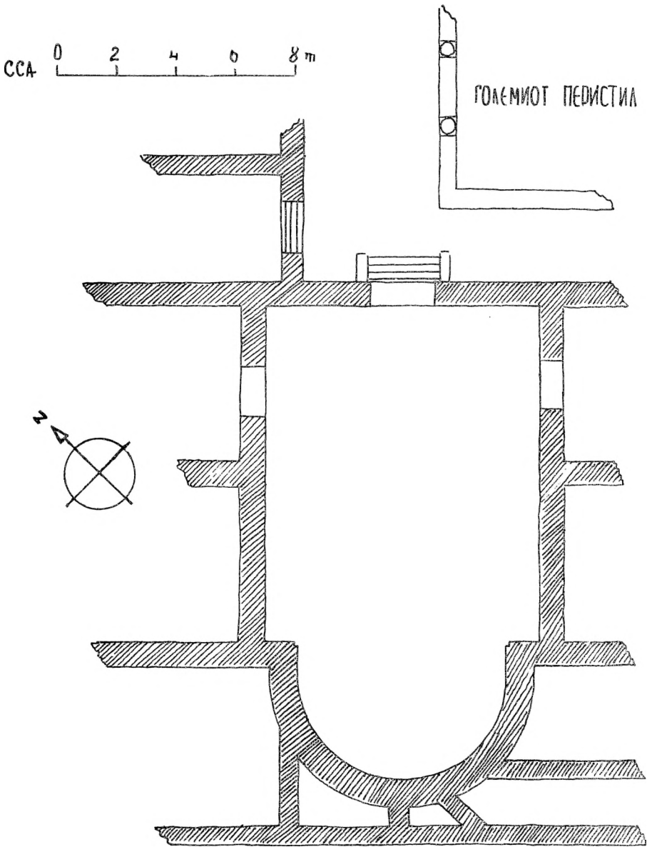
СЛ 10 - ГОЛЕМАТА АПСИДАЛНА ДВОРАНА ВО ПАРТЕНИСОВАТА ПЛАТА ВО СТОБИ СЛОБОДНО МЕРНО ЦАГОЛЕМУВАЊЕ СПОРЕД Б ПЕСТОРОВИЌ
