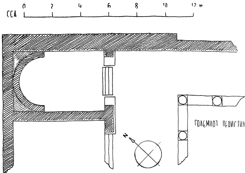
СЛ 11 - МАЛАТА СЕВЕРНА АПСИДАЛНА ОДАЈА ВО ПАРТЕНИОСОВАТА ПАЛАТА ВО СТОБИ СЛОВЕДНО МЕРНО ЦЕГОЛЕМУВАЊЕ СПОРЕД Б ЧЕСТОВОВИЌ И СПОРЕД ДИСПОЗИЦИЈАТА IN SITU
