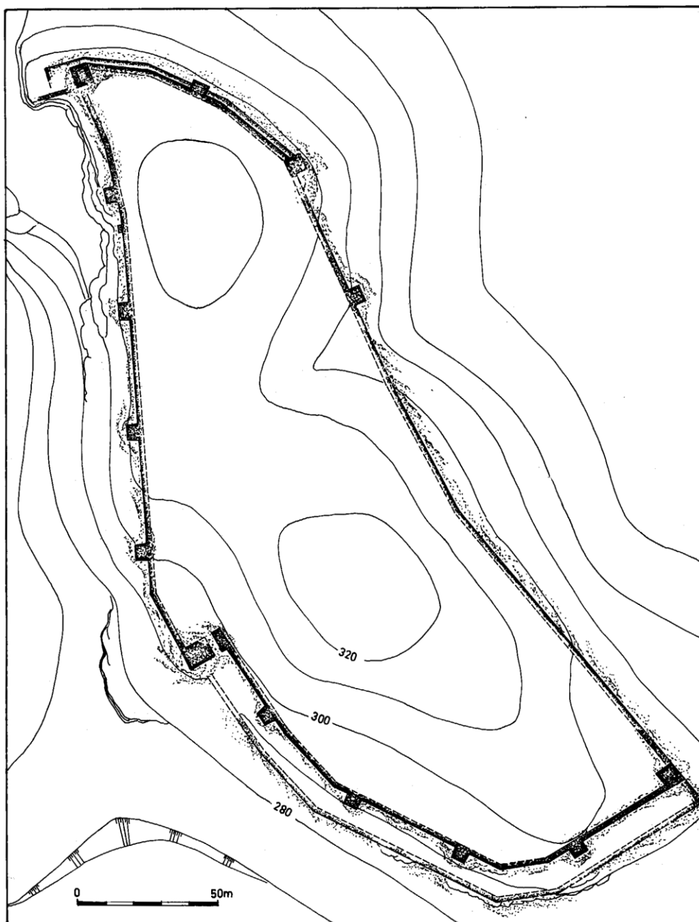
Сл. 36 - Стари Град, Кале, план на И. Микулчиќ
