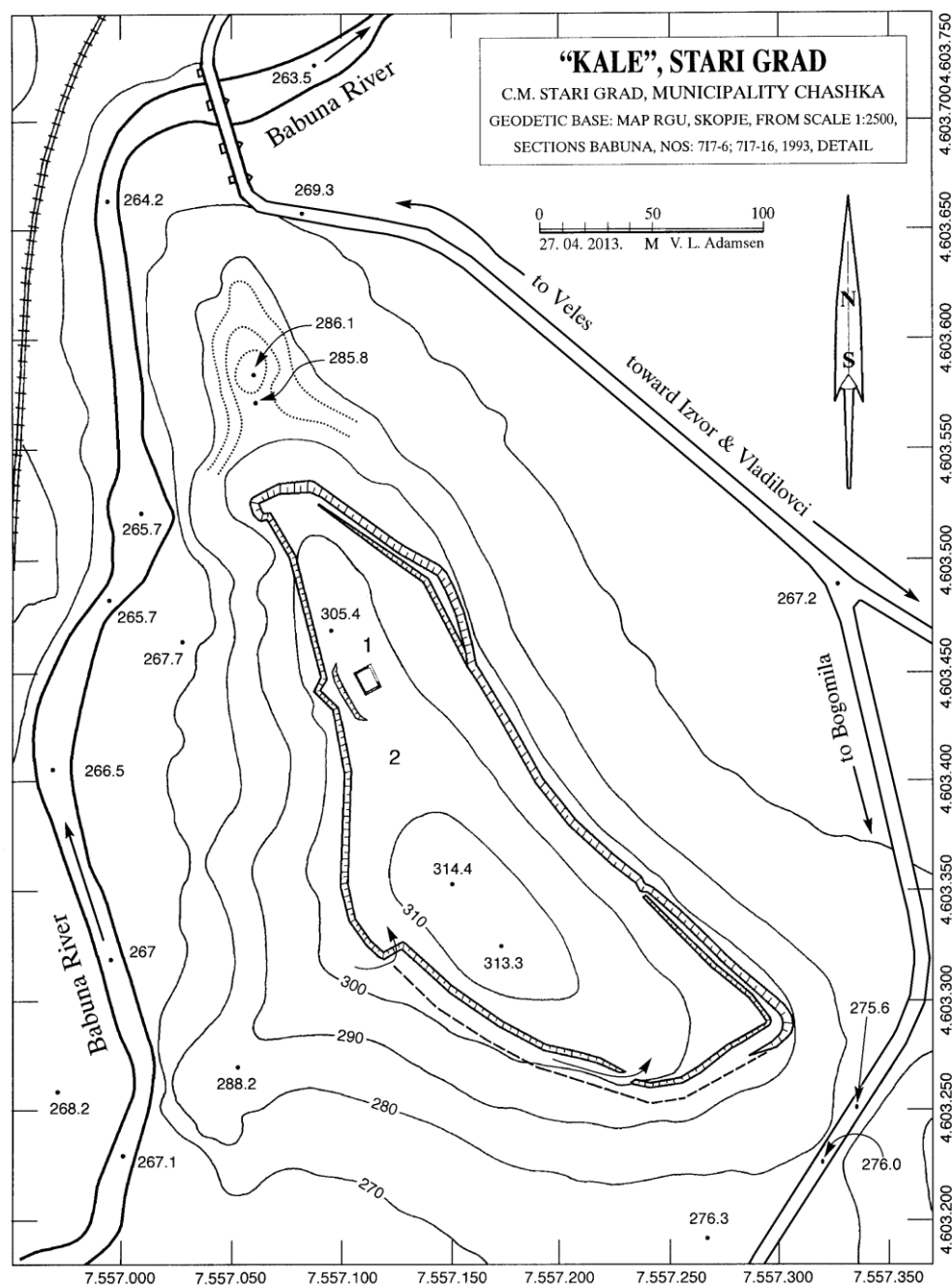
Сл. 37 - Стари Град, Кале, план на В. Л. Адамс
