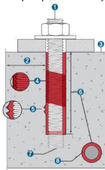
Анкери вградени со хемија
