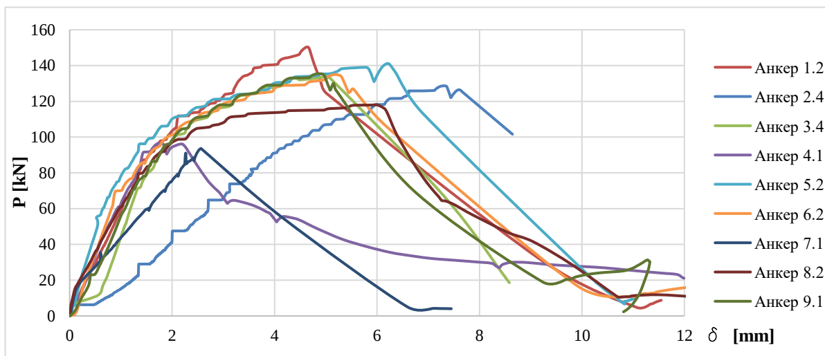
Сл. 6. Карактеристичен сила – поместување дијаграм за испитани механички анкери
