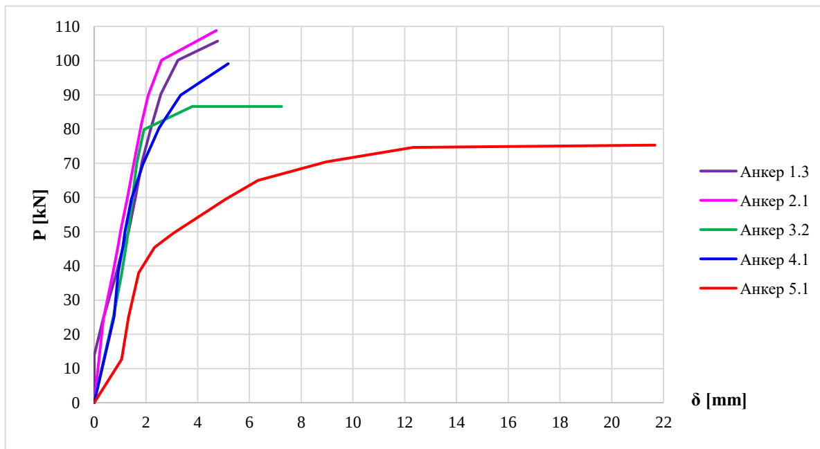
Сл. 8. Карактеристичен сила – поместување дијаграм за испитани механички анкери
