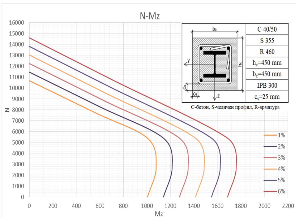
Сл. 3. Дијаграми на интеракција N-Mz за пресек 450x450mm за 1 до 6%
