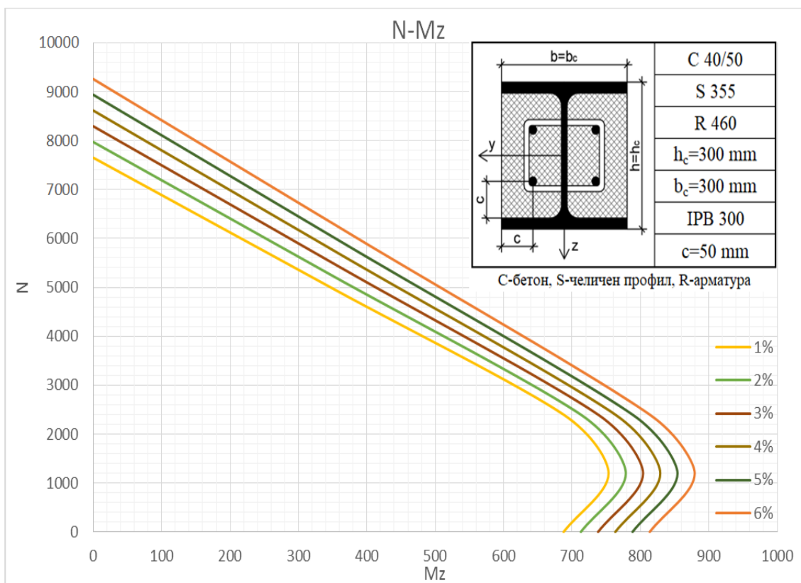
Сл.5. Дијаграми на интеракција N-Mz за пресек 300x300mm за 1 до 6%
