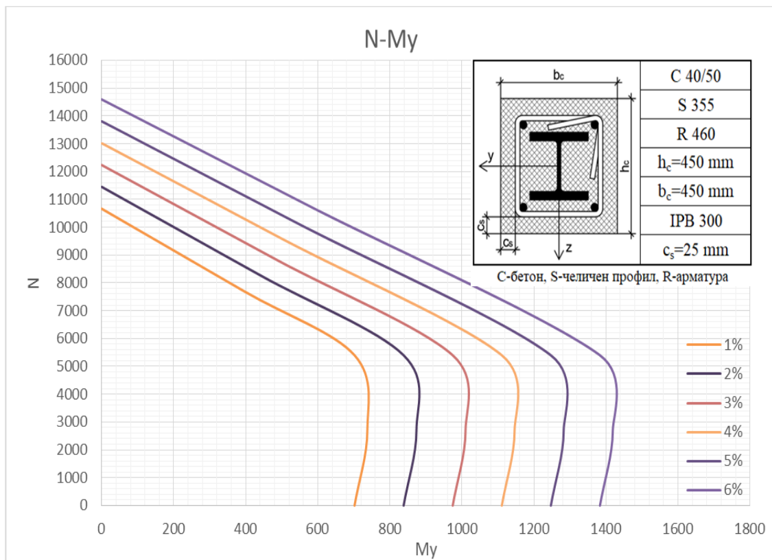
Сл.4. Дијаграми на интеракција N-My за пресек 450x450mm за 1 до 6%
