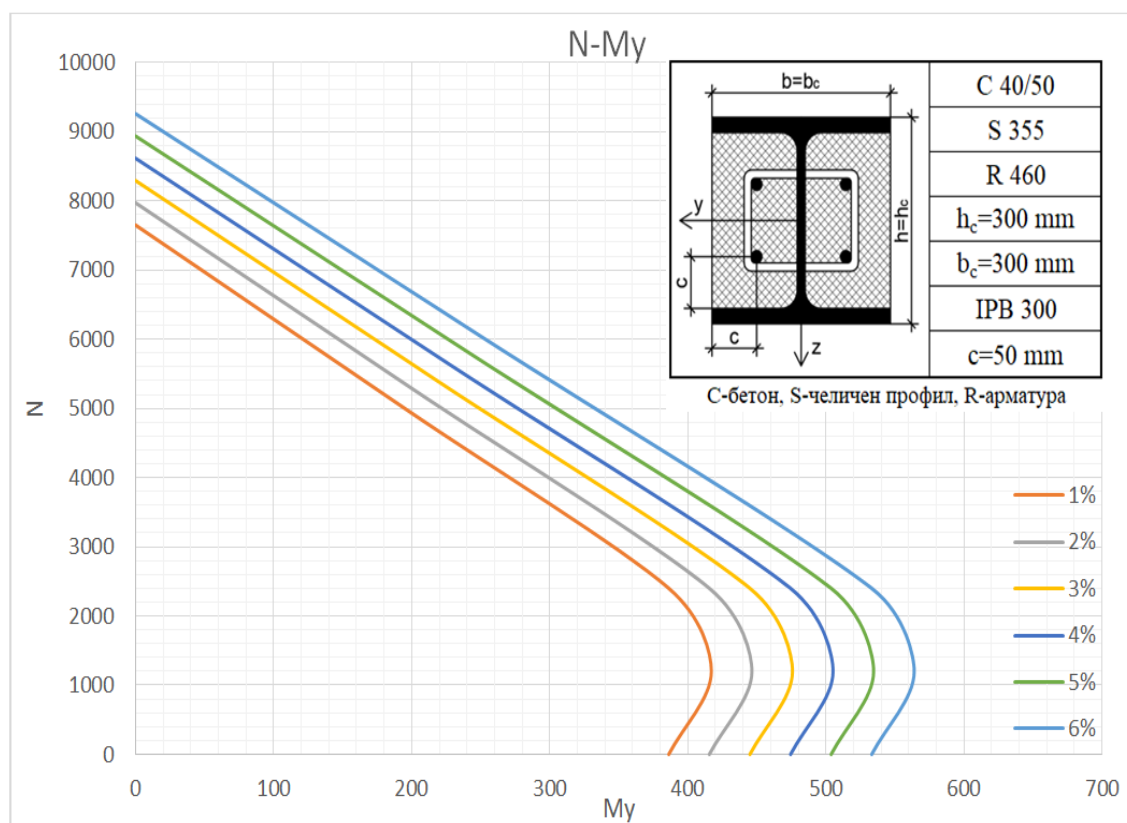
Сл. 6. Дијаграми на интеракција N-My за пресек 300x300mm за 1 до 6%
