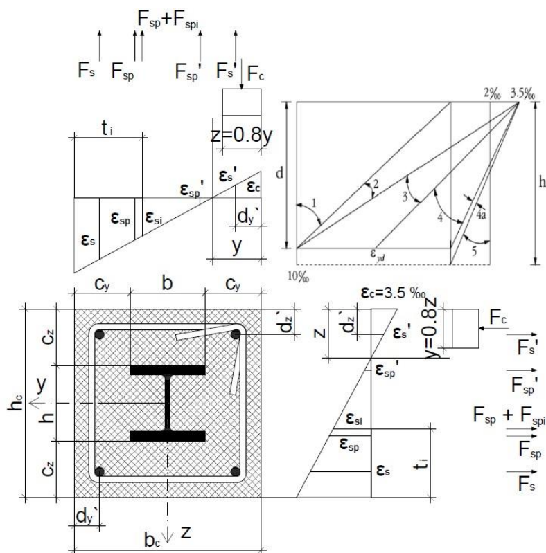
Сл. 1. Распределба на дилатации во попречен пресек
