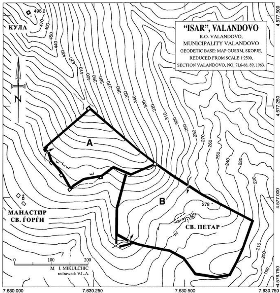
Сл. 21 . План на Исар Валандово А-Акропола, В-Град, според И.М., преработен В.Л.А
