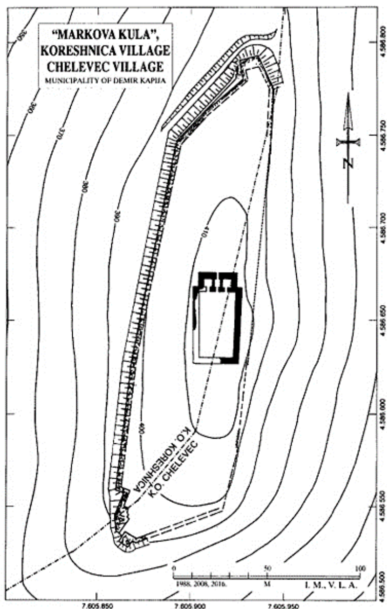
Сл. 38. План на „Маркова Кула“, Корешница, Демир Капија, В.Л.Адамс
