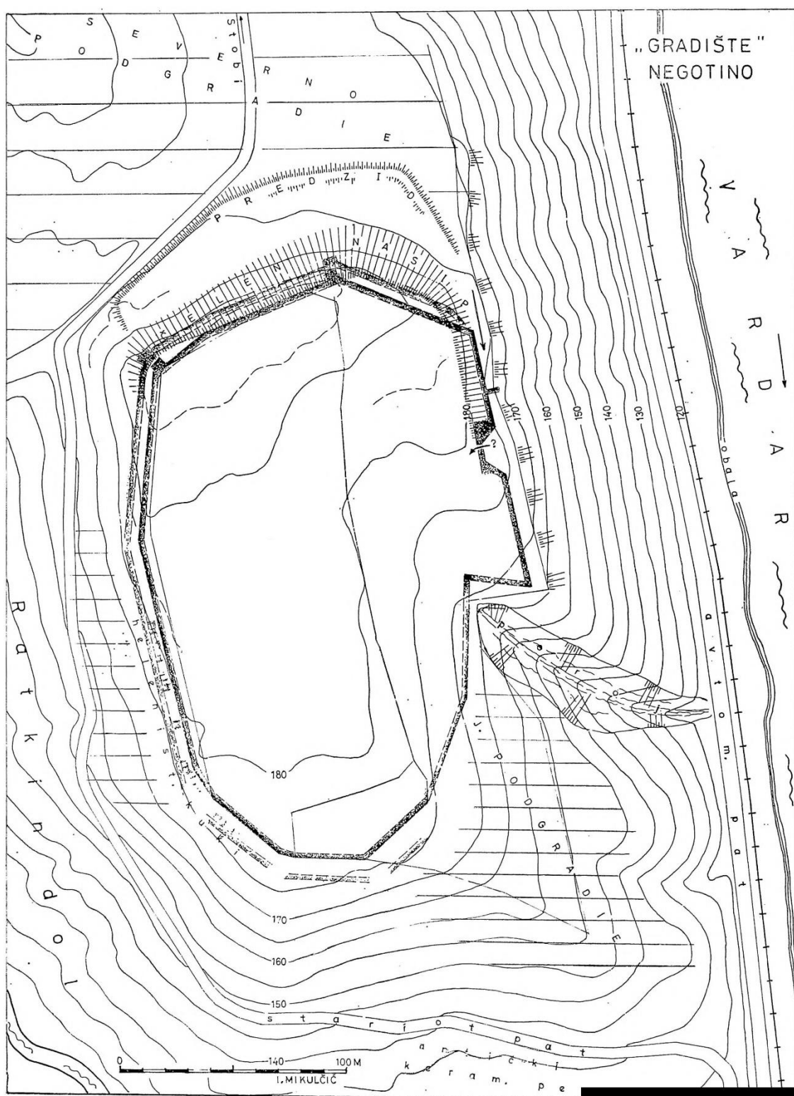
Сл. 25. План на Градиште, Неѓојино (спored И. Микулчиќ)
