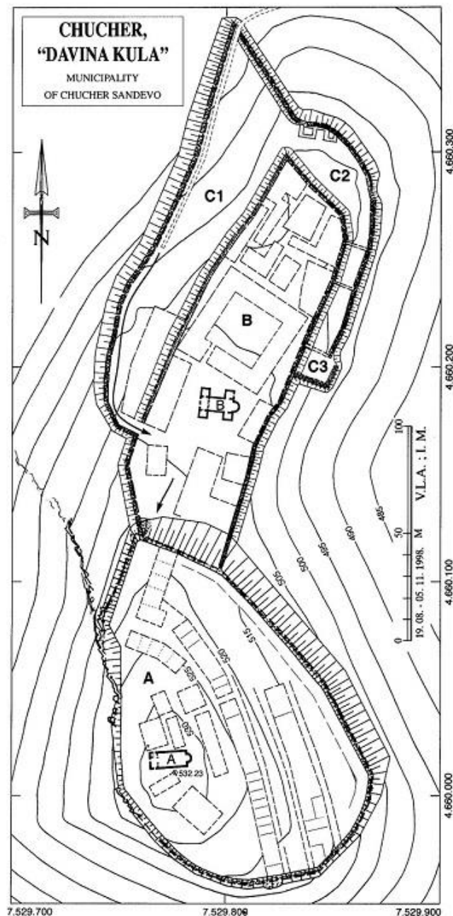
Сл. 24. Давина Кула план- В. Л. Адамс и И. Микулчиќ
