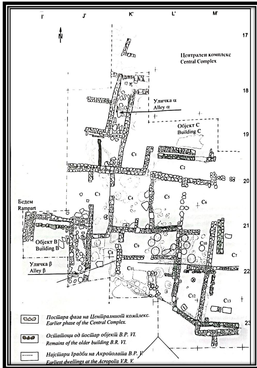
Сл. 13. План на зградби на Акрополата (според Д. Митревски)
