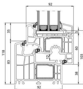
Слика 23 PVC Salamander bluevolution 92
