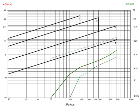
Дијаграм 9. Пропустливост на воздух – подгрупа 9/2
