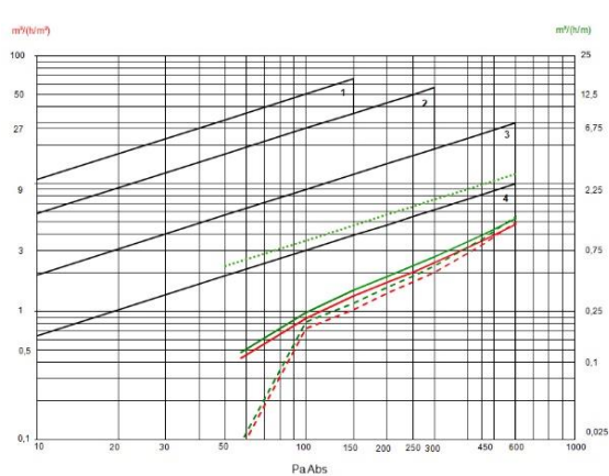
Дијаграм 34. Пропустливост на воздух – подгрупа 6/6
