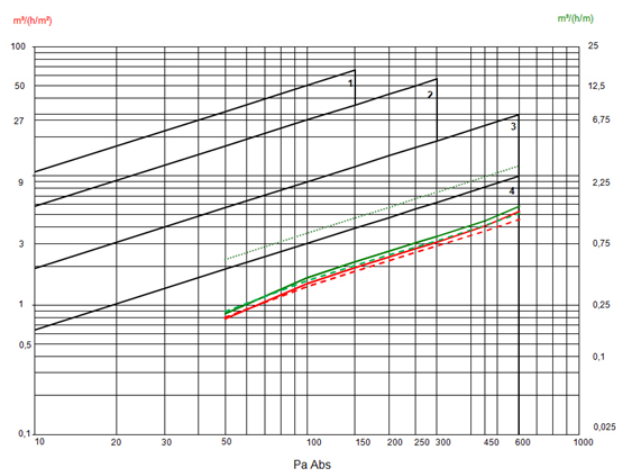
Дијаграм 4. Пропустливост на воздух – подгрупа 4/2
