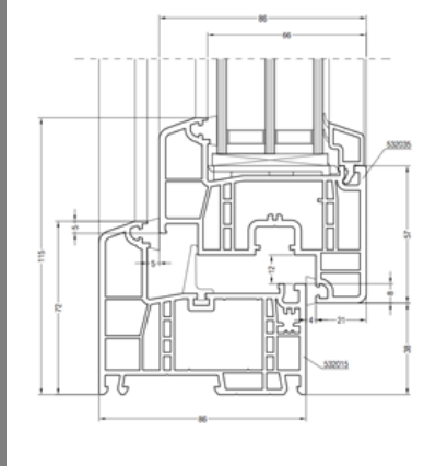
Група 4/7 Прозорци со димензија 800/2000mm PVC профил REHAU GENEО [115]
