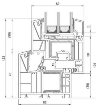
Слика 22 Aluplast energeto 8000
