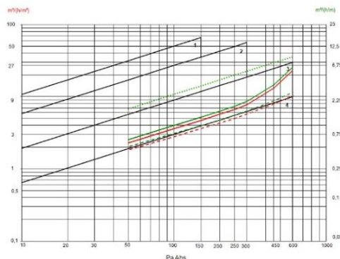
Дијаграм 19. Пропустливост на воздух – група 4/4
