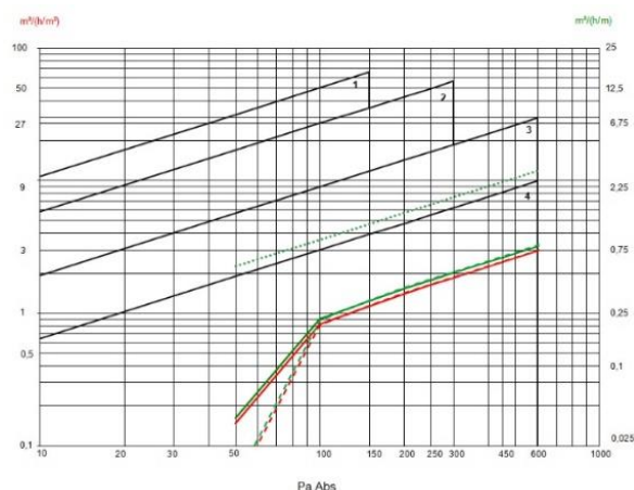
Дијаграм 37. Пропустливост на воздух – подгрупа 9/6
