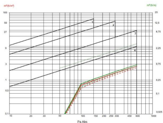
Дијаграм 29. Пропустливост на воздух – подгрупа 1/6
