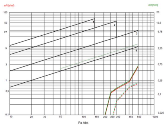
Дијаграм 5. Пропустливост на воздух – подгрупа 5/2
