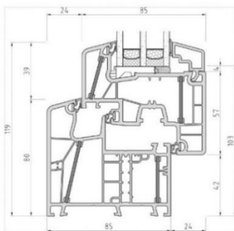
Слика 21 Salamander greenevolution
