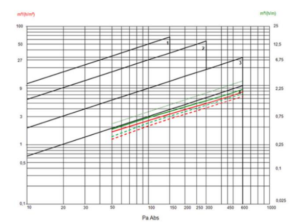
Дијаграм 8. Пропустливост на воздух – подгрупа 8/2
