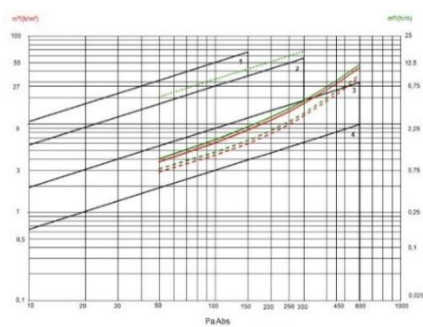
Дијаграм 14. Пропустливост на воздух – група 2/3 (алуминиумски профил)
