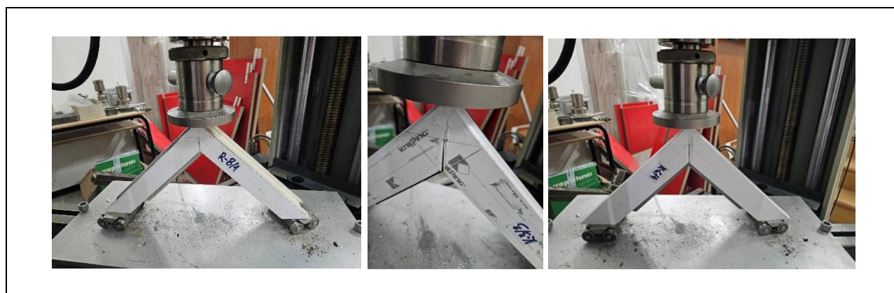
Слика 33 Делување на сила кај примероци од група крило
