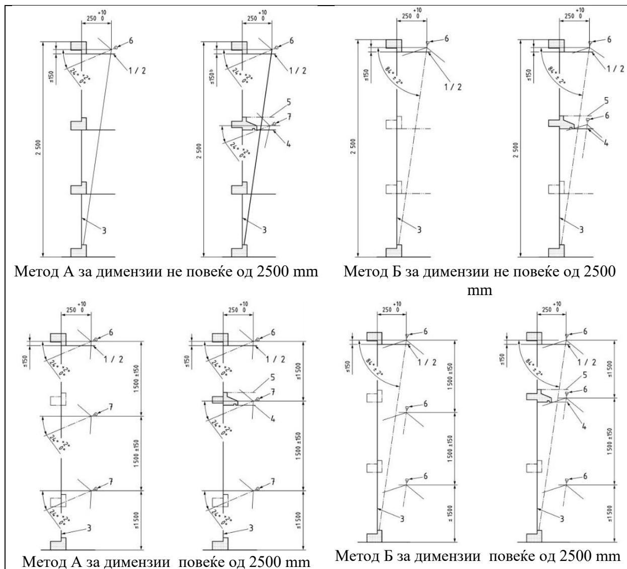
Слика 10 Распоред на прскалки согласно димензијата на прозорецот
