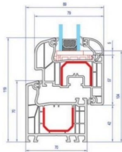
Слика 26 Пресек од профил на рамка и крило
