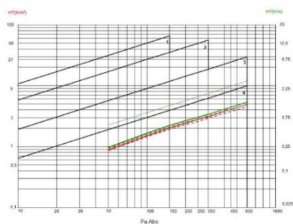
Дијаграм 13. Пропустливост на воздух – група 1/3 (ПВЦ профил)
