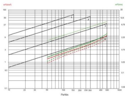
Дијаграм 15. Пропустливост на воздух – група 3/3 (дрвен профил)
