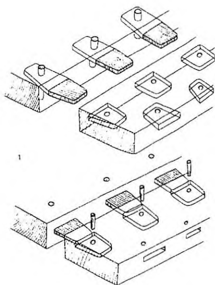
сл. 3.1. Зацврстување на штиците од опшивката со помош на отвори (L. Casson, The Ancient Mariners , second ed., Princeton 1991, 28)
