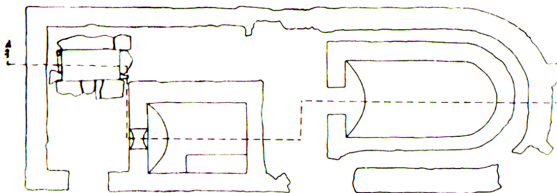
Слика 48. План на мартириумот во Бањица (АМК,2012)
