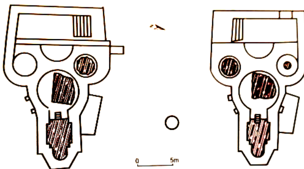
Слика 21. План на прстеновидните градби (F. Peja, B. Rraci, A. Hajdari: Castle of Harilaq, 2012)
