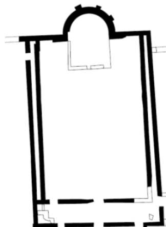
Слика 42. План на Епископската базилика во Улпијана (Brochure, 2016)
