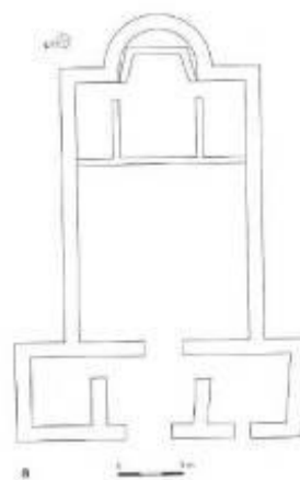
Слика 9. План на црквата во Кориша (AMP, 2006)
