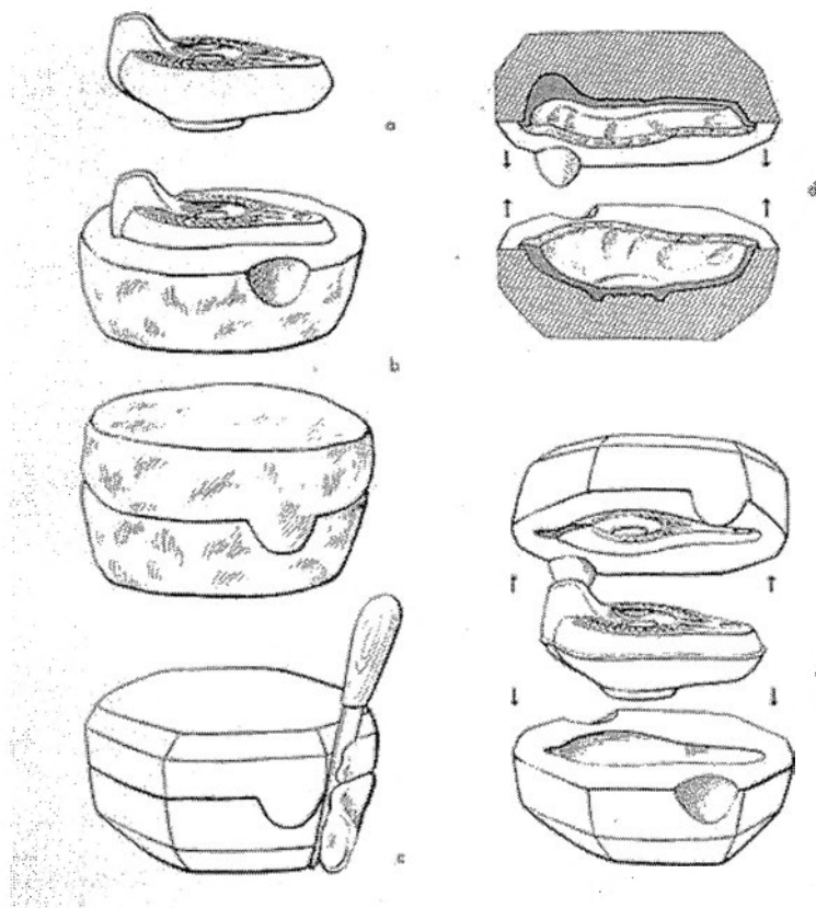
Слика 5. Изработка на калап од светилка. 49
