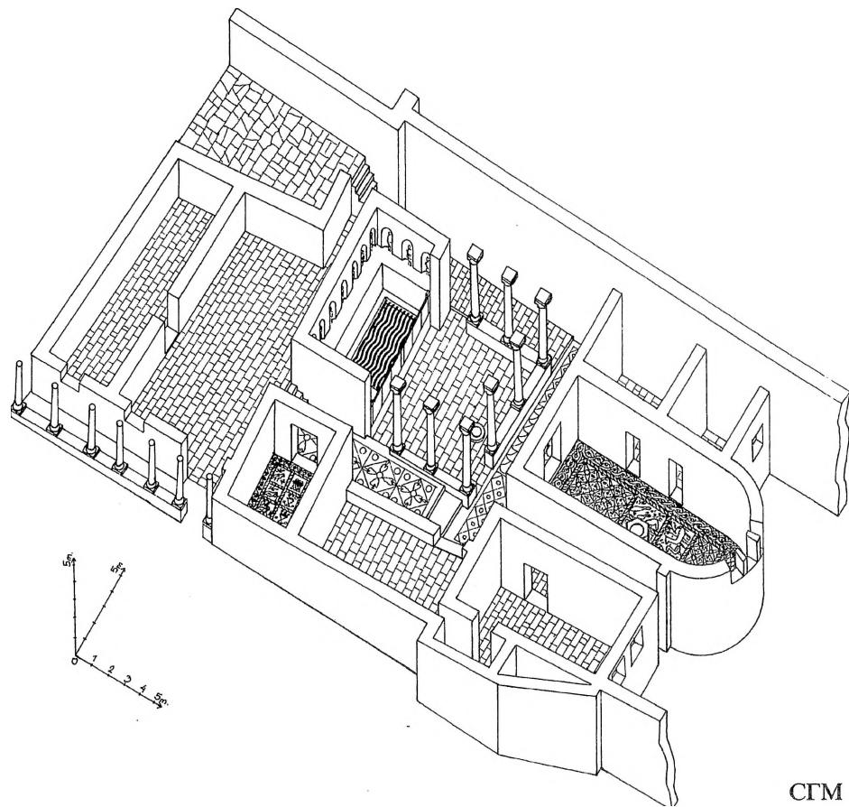
Сл. 9 Стоби. Т.н. Куќа на Полихарм. Аксонометрија на репрезентативната фаза
