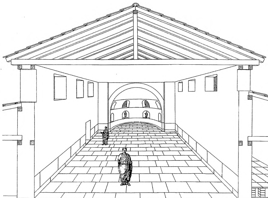
Сл.13 Стоби. Т.н. Домус Фулоника. Голем триклиниум. Можна реконструкција. СГМ.
