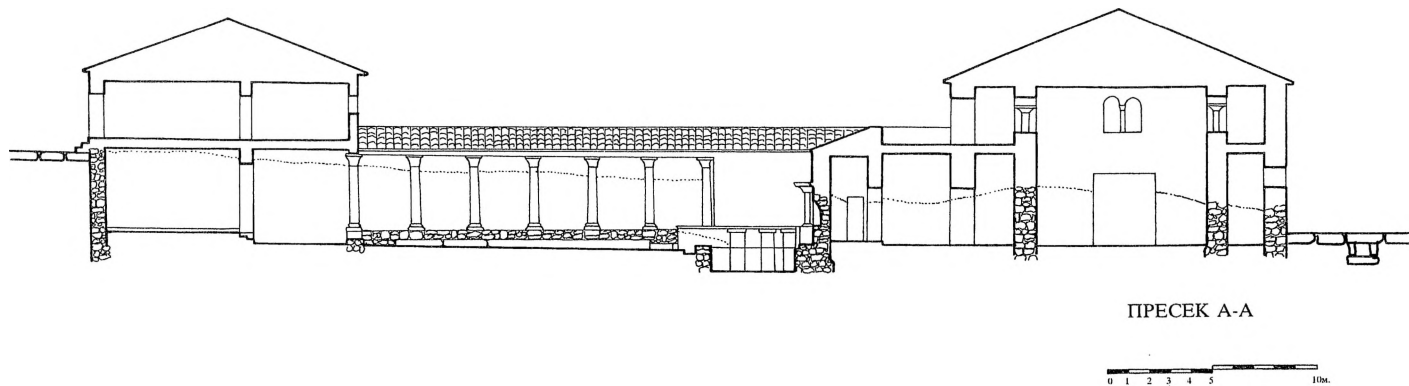
Сл. 3 Стоби. Т.н. Куќа на Партениј. Северен репрезентативен дел, пресек. (Реконструкција според Б.Несторовиќ).
