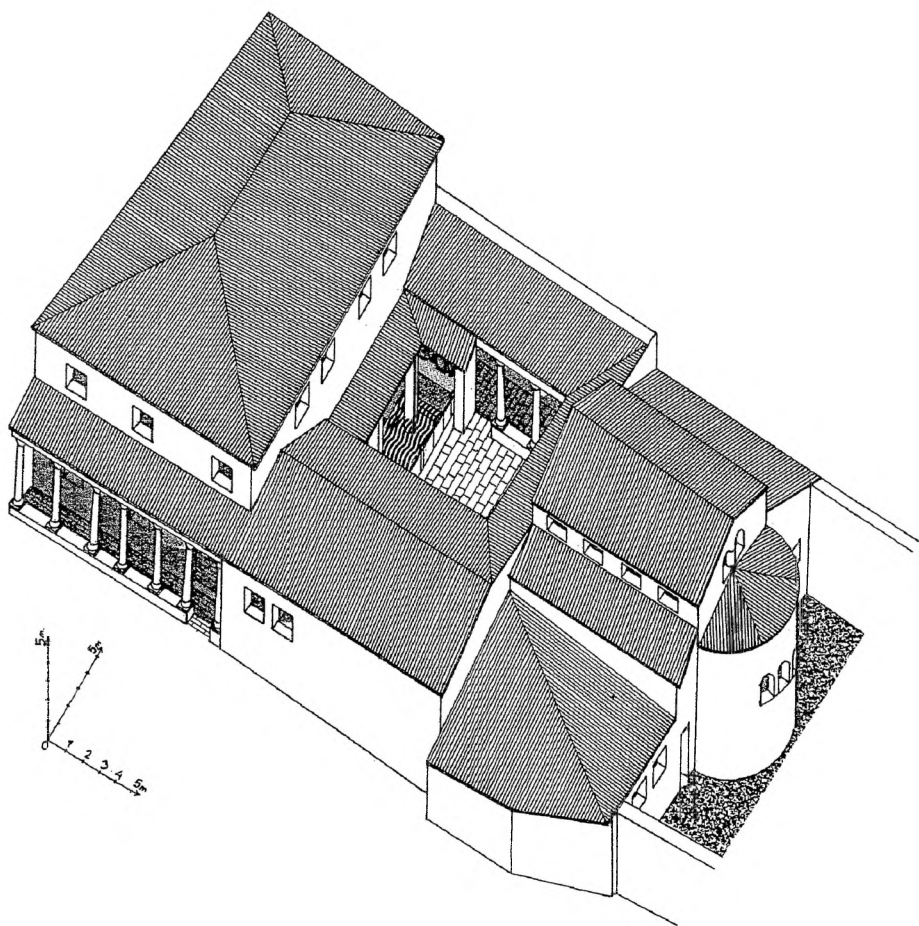
Сл. 10 Стоби. Т.н. Куќа на Полихарм. Можна реконструкција. СГМ
