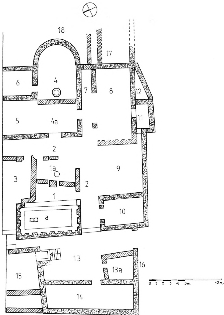
Сл. 8 Стоби. Т.н. Куќа на Полихарм. Основа со преградувања од доцниот 4.-5. век (шрафирано).
