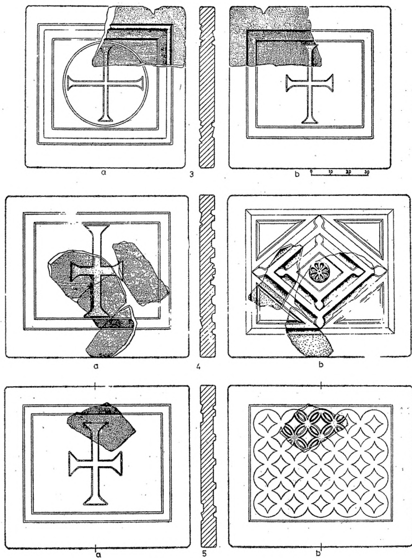
сл. 3—5 Давина, Чучер, базилика В, делови од паранетни плочи.
