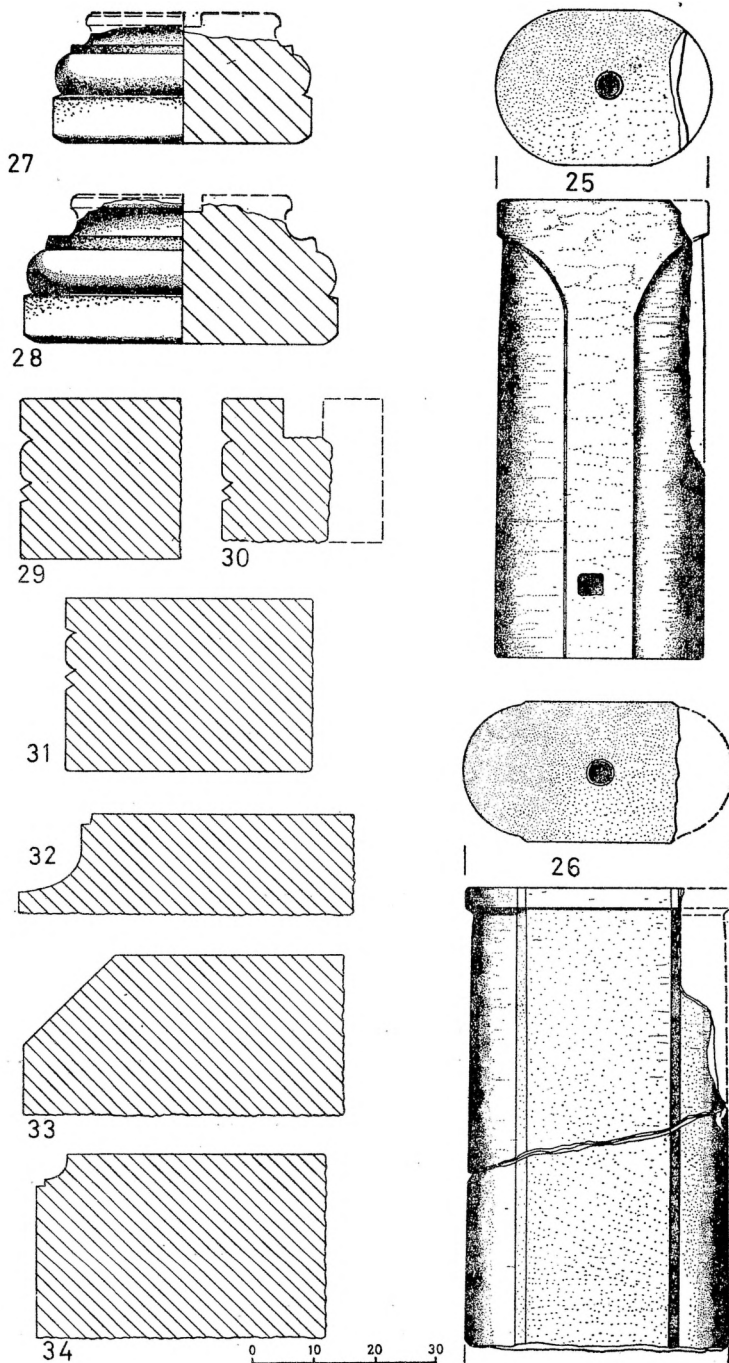
Св. Спас, Матка, ранохристијански менои (сл. 23, 25), јонски базили (сл. 27, )28 раноримски архитравни греди и постаменти (пресеци; сл. 29—34).
